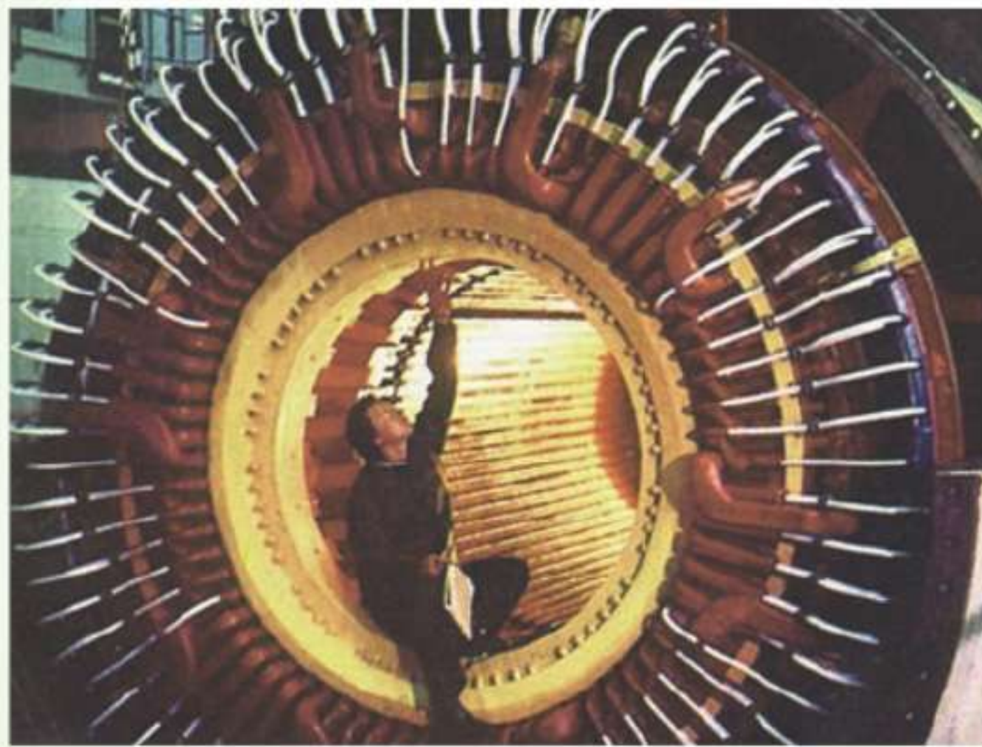
Сборка генератора на заводе «Электросила»
